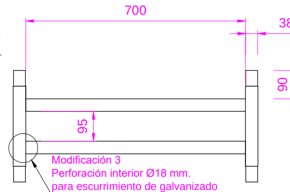
DETALLE CORTE A-A'
