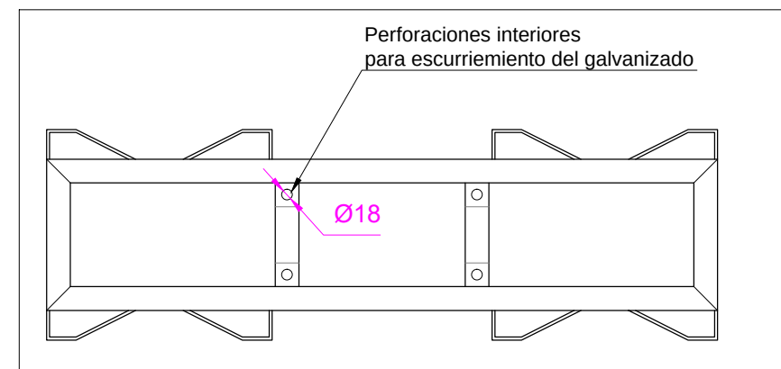
DETALLE CORTE B-B'
