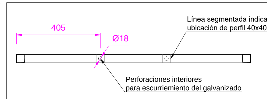
DETALLE CORTE B-B'
